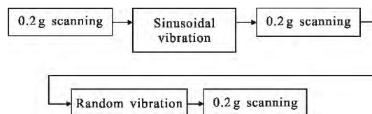
图 3 星敏传感器支架力学试验顺序
