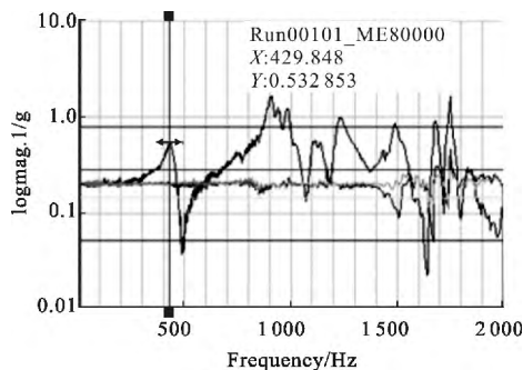
图 4 星敏传感器组件力学 X 向 0.2 g 特征试验曲线
