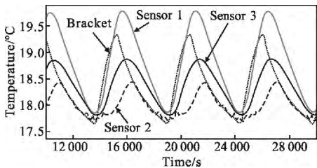
图 7 高温瞬态工况温度变化
