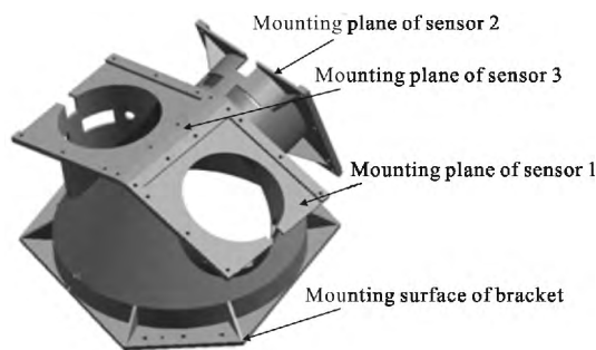
图 1 星敏感器支架结构图
