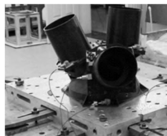
图 2 星敏传感器组件力学试验状态图
