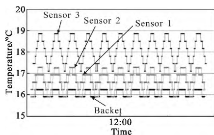
图 8 在轨温度曲线
