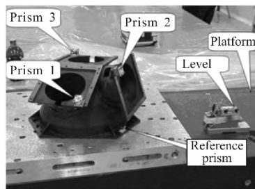
图 5 星敏传感器支架立方棱镜位置图
