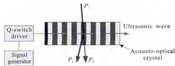
图 1 声光 Q 开关工作原理图
