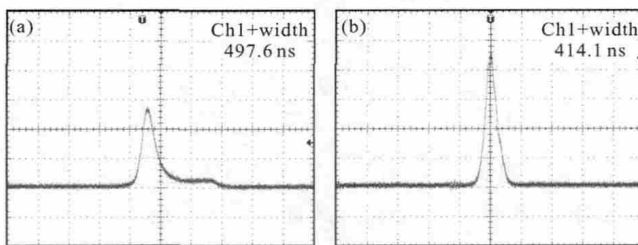
图 4 占空比为 80% 和 90% 时的激光单脉冲波形
