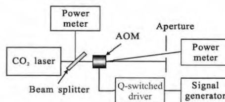
图 3 衍射效率测量原理图
