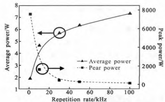
图 6 平均功率和峰值功率随重复频率变化曲线
