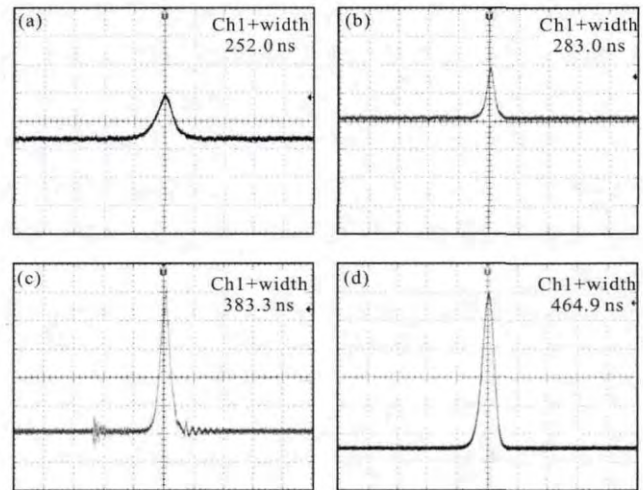
图 5 重复频率为 1 kHz、10 kHz、30 kHz 和 100 kHz 时的激光单脉冲波形
