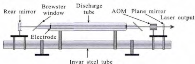
图 2 声光调 Q CO 2 激光器实验装置图
