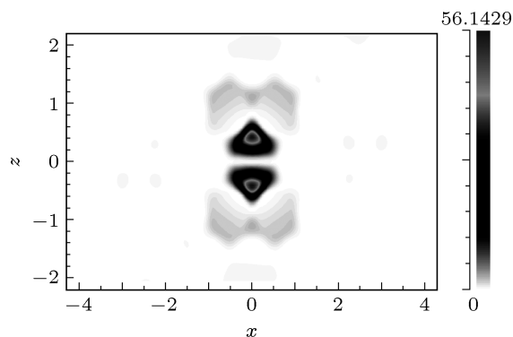
图 4 微腔模式的模式场
