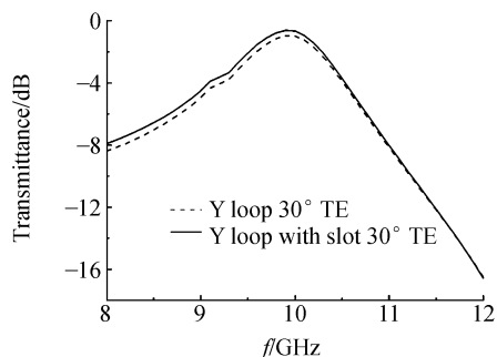
图7 30 TE波入射情况下两种结构透射比对照
