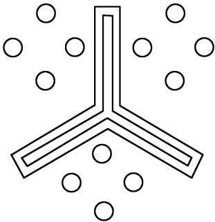
图 5 设置圆孔的 Y 环单元 Fig. 5 Y loop with circle slot
