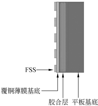
图 1 FSS 的分析模型 Fig.1 FSS model
