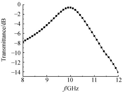
图 3 正入射下 Y 环单元 FSS 的频率响应曲线 Fig.3 Curve of frequency response under perpendicular incidence
