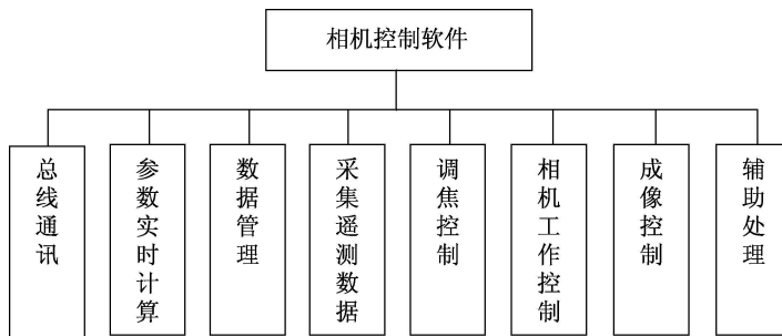
图 1 相机控制软件系统功能框图
