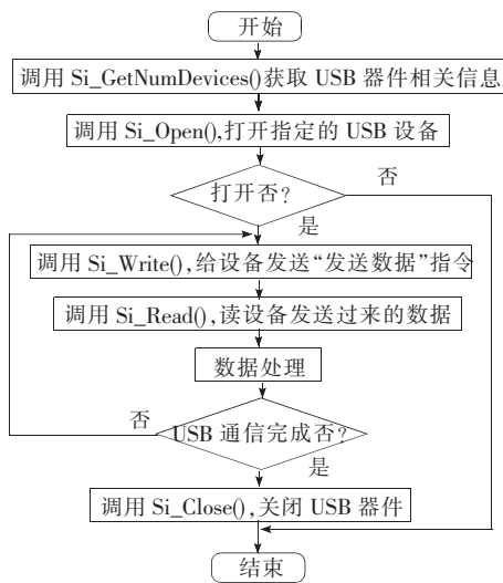
图 3 PC 应用程序流程图
