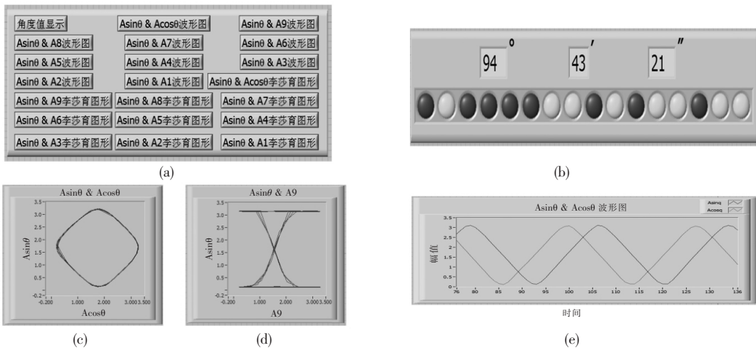
图 5 系统界面。(a)菜单;(b)角度显示;(c) Asin\theta & Acos\theta 李莎育图形;(d) Asin\theta & A9 李莎育图形;(e) Asin\theta & Acos\theta 波形图。
