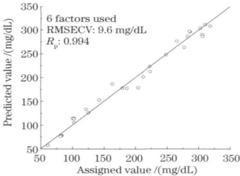
图 5 模拟组织液光谱的定标结果
