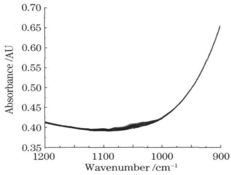
图 3 模拟组织液的原始光谱 Fig.3 Raw ATR-FTIR spectra of simulated interstitial fluids 一共得到 30 条光谱, 其中一志愿者的手指光谱如图 4所示。
