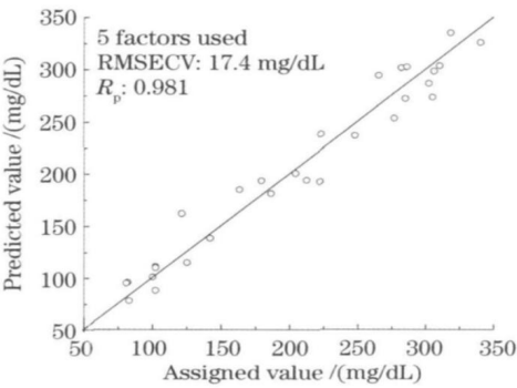
图 7 手指与模拟组织液加和光谱的定标结果
