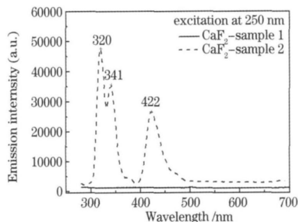
图 5 CaF 2 衬底的光致发光光谱
