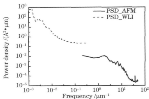
图 4 CaF 2 衬底表面的一维 PSD 函数
