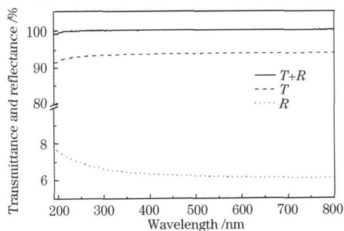
图 1 \text{CaF}_2 衬底的透射和反射测量光谱
