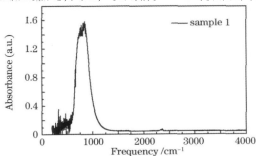
图 6 CaF 2 衬底的 FTIR 光谱
