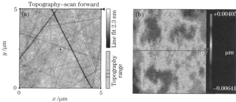
图 3 CaF 2 衬底表面粗糙度测量结果。(a) 原子力显微镜(5 μm × 5 μm) 测量结果; (b) 白光干涉仪(0.94 mm × 0.70 mm) 测量结果
