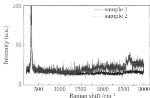
图 7 CaF 2 衬底的拉曼光谱
