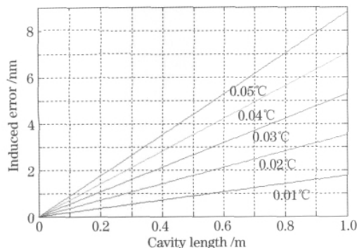
图 2 温度变化引入的测量误差
