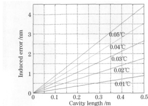
图 6 温度径向梯度引入的测量误差
