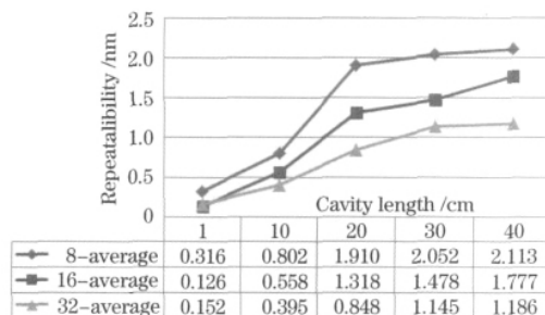
图 9 不同腔长测量结果偏差
