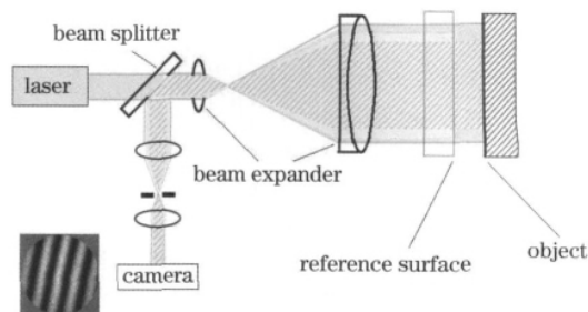
图 1 Fizeau 干涉仪原理示意图
