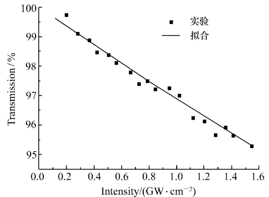
图 2 偶氮透过率曲线
