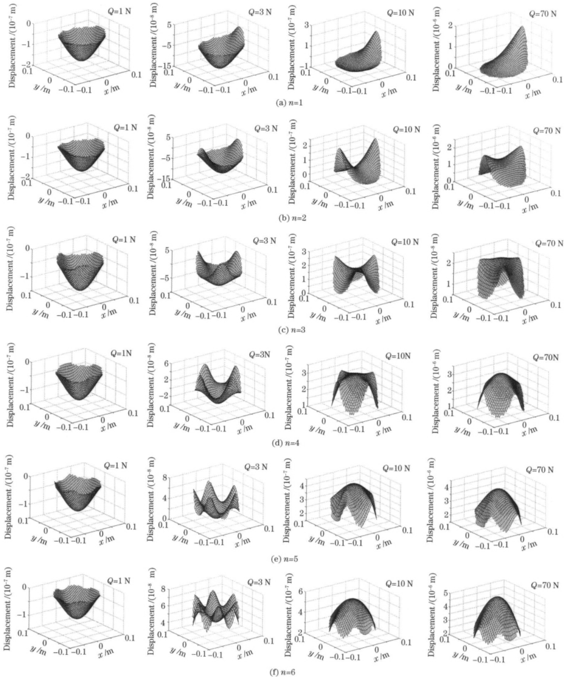
图 6 有效口径内镜片的挠度变化 Fig. 6 Deflection of lens in effective aperture
