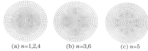
图 5 模型的网格划分 Fig. 5 Meshes of model
