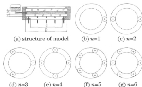
图 4 主动液体透镜的分析模型
