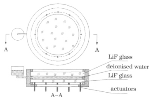
图 1 主动液体透镜示意图
