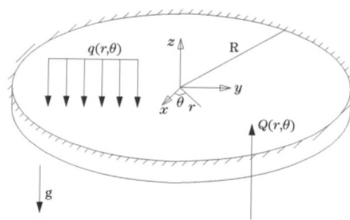
图 2 下层玻璃薄板的物理模型
