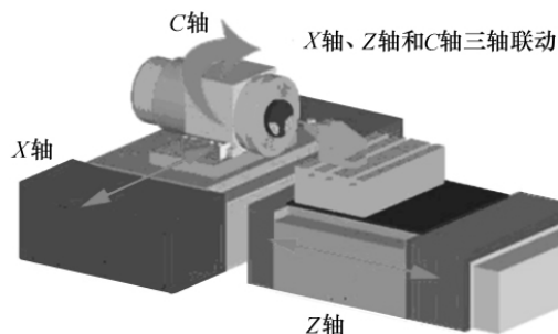
图18 慢刀伺服系统示意图
