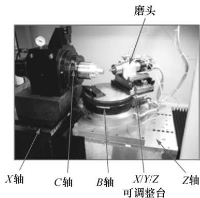
图5 配有 XZCB 和磨头的金刚石机床
