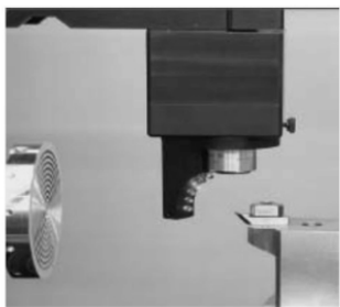
图 11 光学对刀装置
