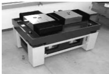
图6 Nanotech 450UPL 的床身与隔振系统
