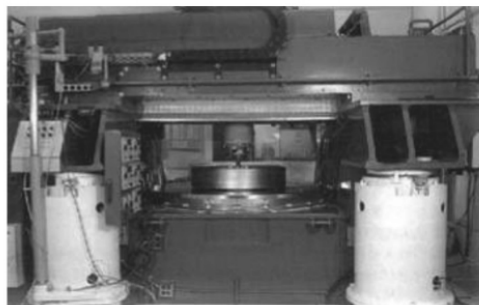
图1 美国的LODTM立式金刚石车床
