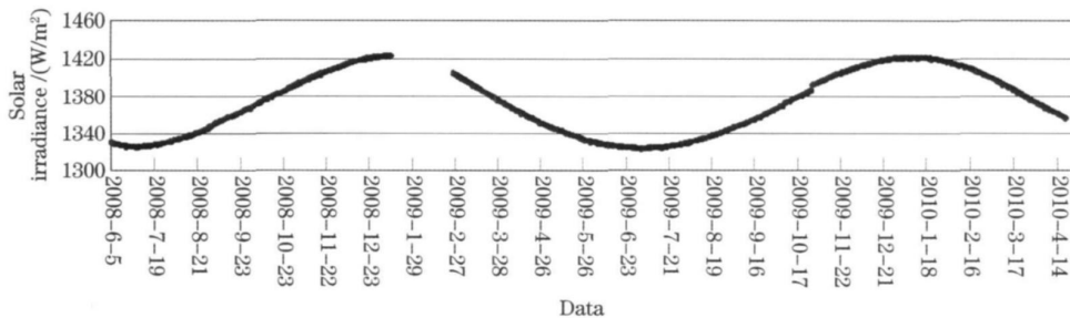
图 2 太阳辐射照度原始值
