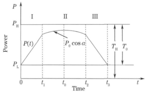
图 6 绝对辐射计接收的辐射功率示意图
