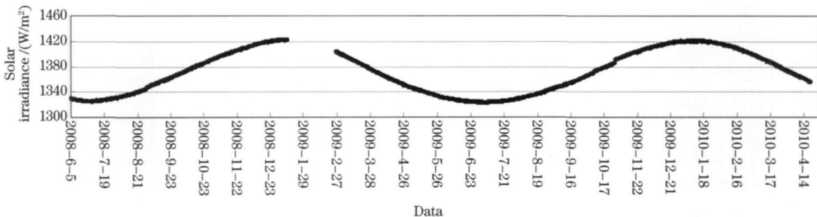
图 10 太阳辐射照度值
