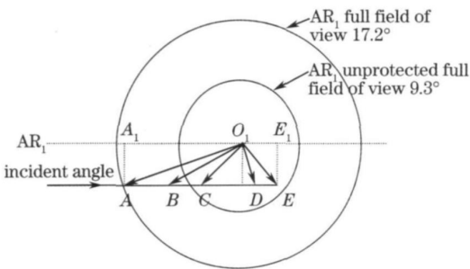
图 5 辐射计视场内入射光与辐射计光轴的夹角示意图
