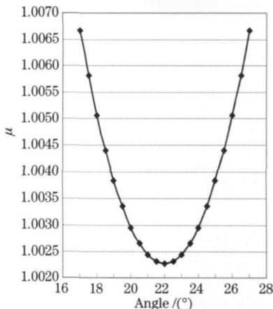
图 9 角度修正系数的拟合曲线
