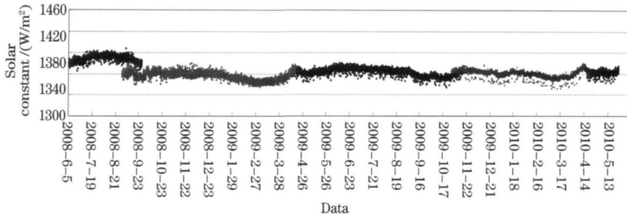
图 11 太阳常数值
