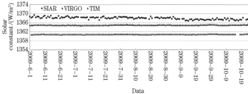
图 12 FY-3 测得的太阳常数同国外同期数据比对
