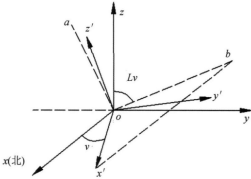
图 3 经轴误差示意图
