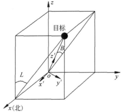
图 2 跟踪状态坐标系示意图
