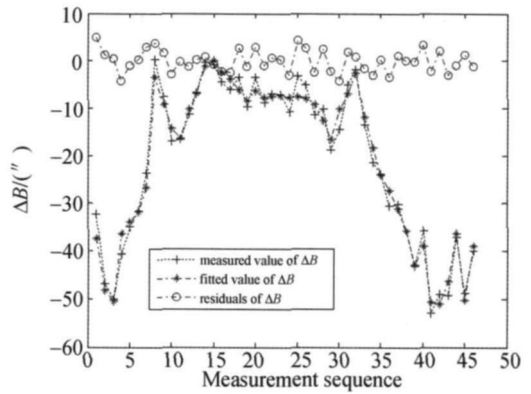
图 5 纬角方向指向误差曲线
