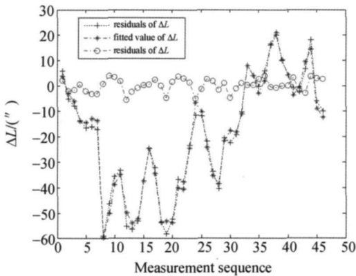
图 4 经角方向指向误差曲线
