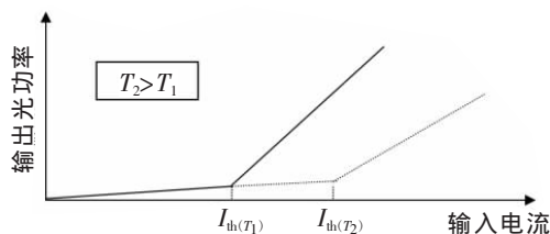
图 1 半导体激光器的光输出功率-输入电流关系
