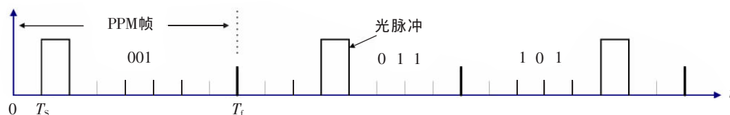
图3 3比特PPM调制光脉冲序列示意图
