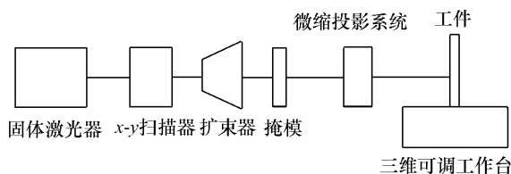
图1 光束扫描宽化掩模投影激光微加工原理示意图
