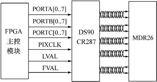
图 3 Camera Link 接口电路 Fig.3 Camera Link interface circuit
