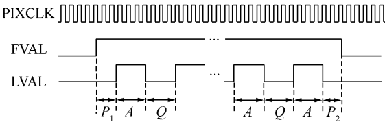
图 5 视频同步控制信号时序
