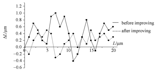
图 6 20 mm 周期内的测量误差曲线
