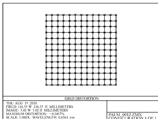
图10 双远心光学系统的网格畸变
