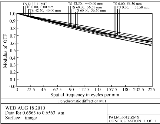
图 9 双远心光学系统的 MTF 曲线
