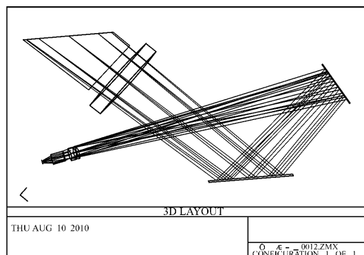
图3 全树脂材料的光学系统图
