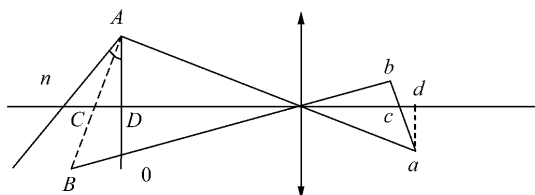
图1 倾斜物面成像的理想光路图
