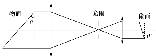
图2 双远心光路图
