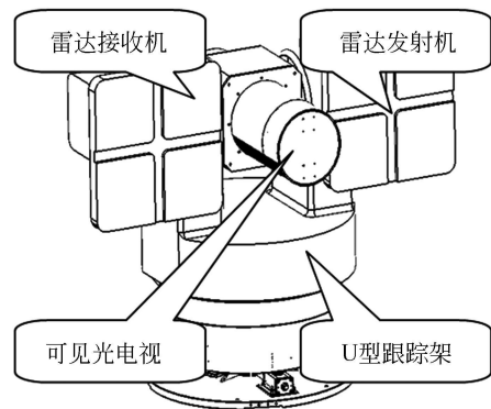
图 1 系统组成结构图
