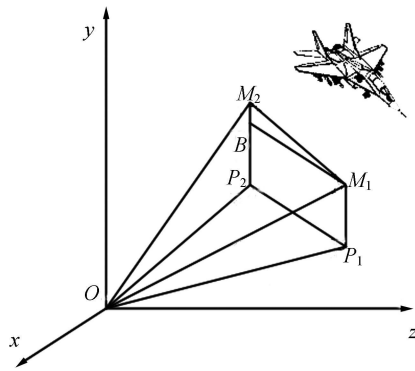
图 2 测站坐标系目标特征点的位置关系
